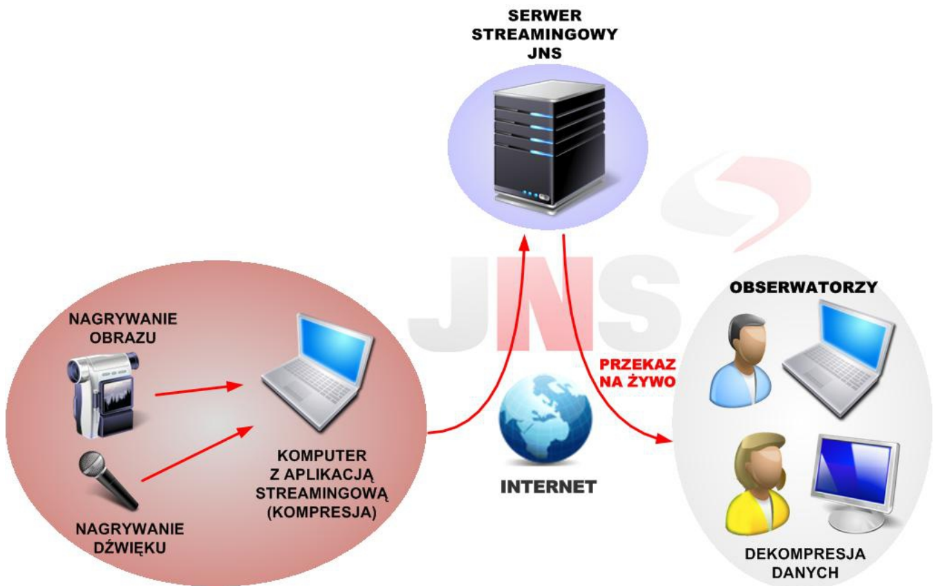
Rys.1 Schemat działania Systemu Live Streaming.
